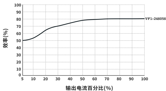
效率 VS 输出负载曲线图 (Vin=24V)
