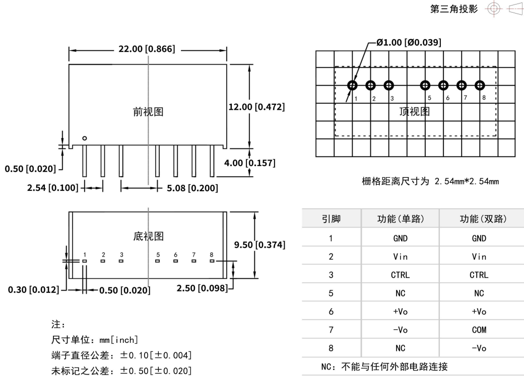
VB1-xxDxxS 外观尺寸与建议刷版图
