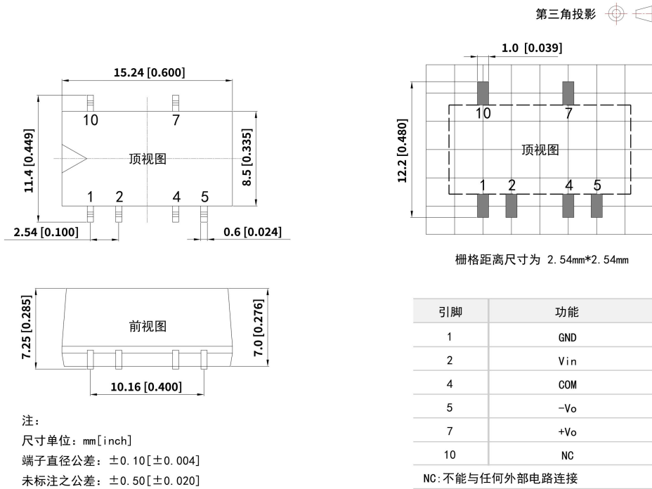
DF2-xxDxxXT 外观尺寸与建议刷版图
