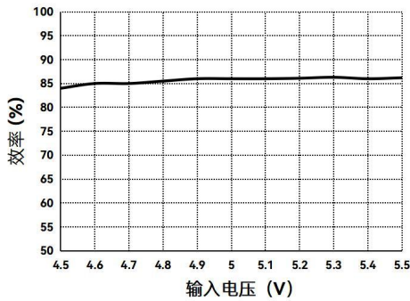
效率 VS 输入电压曲线图 (满载、DF2-05D05XT)
