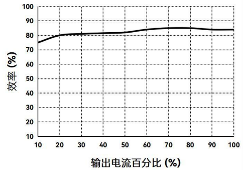
效率 VS 输出负载曲线图 (Vin=12V、DF2-05D05XT)
