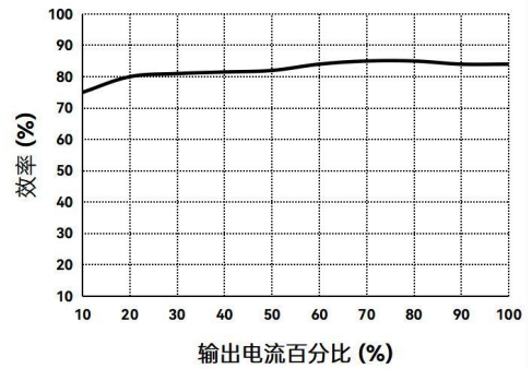
效率 VS 输出负载曲线图 (Vin=5V, DB2-05D05XT)
