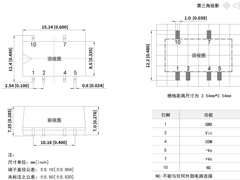
DB2-xxDxxXT 外观尺寸与建议刷版图
