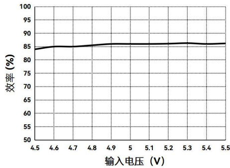
效率 VS 输入电压曲线图 (满载, DB2-05D05XT)
