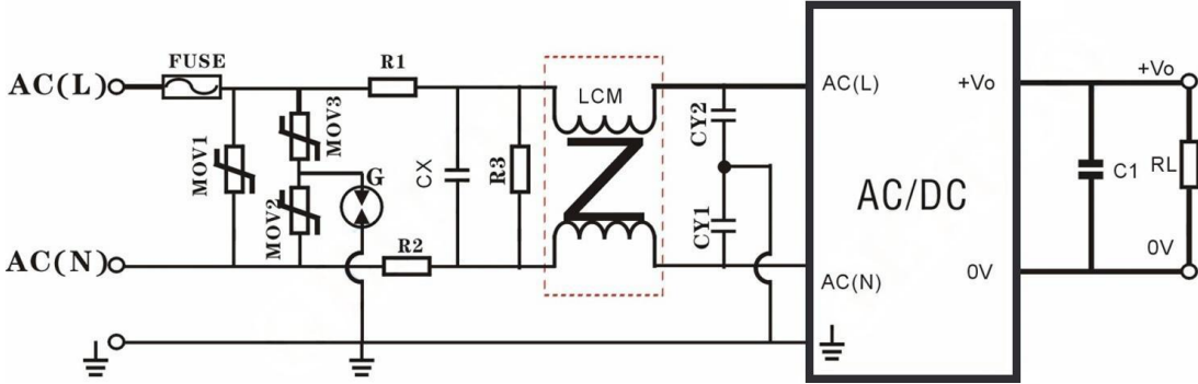
EMC 解决方案-推荐电路
